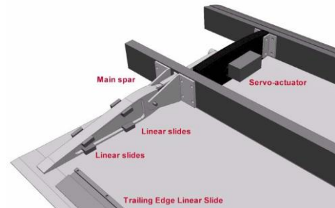
Fig. 7. Rotating rib concept of Politecnico di Milano [12].
