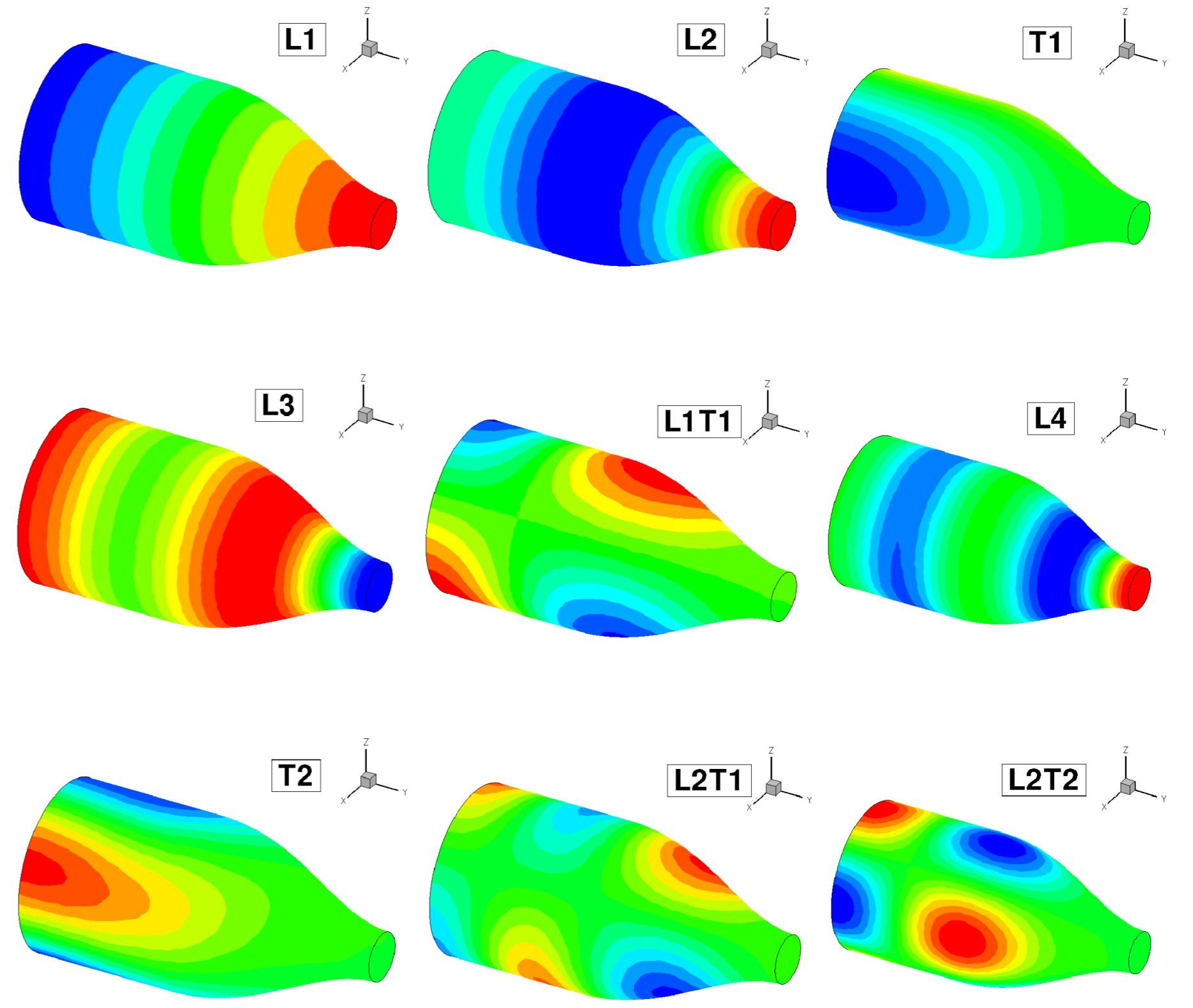
Roket yanma odası modları
