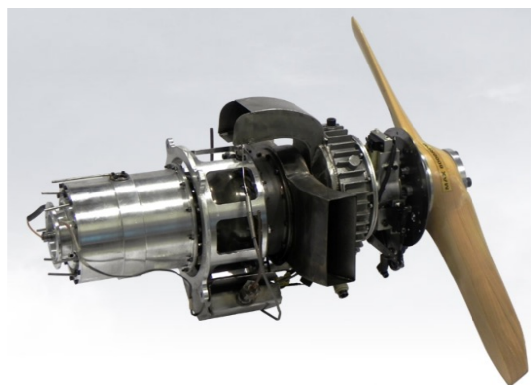
TEİ-TP38 Turboprop motoru
