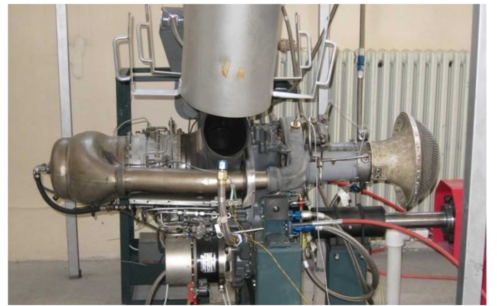
TEİ-TJ300 Turbojet motoru
